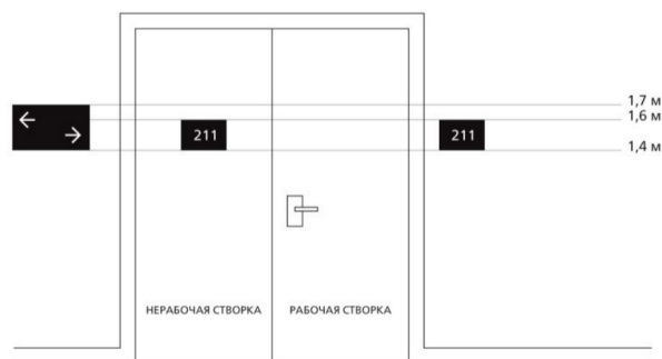
Рисунок 8 — Вариант размещения информации на нерабочих створках дверей
